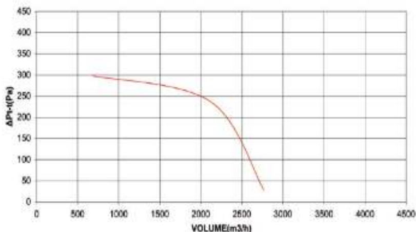
Φ200-0.5HP-1450RPM
