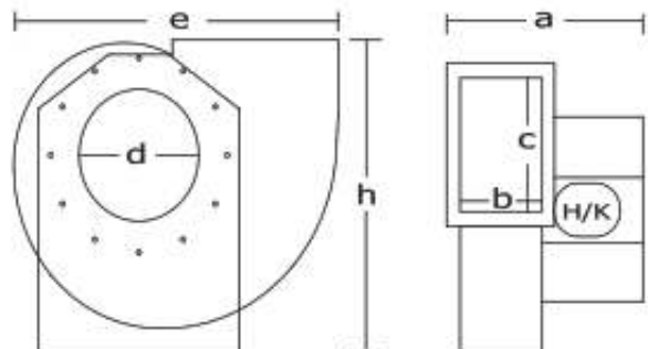
Φ200-0.5HP-1450RPM
